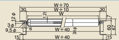
TRC-3812
