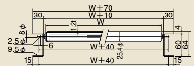
TRC-2508
